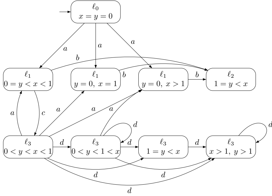
Fig. 5: A region automaton
